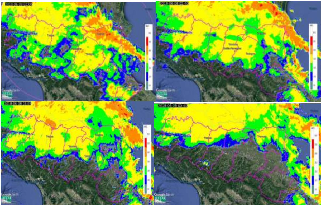
Figura 14. Mappe di riflettività del 08/06/2018 alle 02:00 UTC (in alto a sinistra), alle 02:40 UTC (in alto a destra) alle 03:05 UTC (in basso a sinistra), alle 03:40 UTC (in basso a destra).
