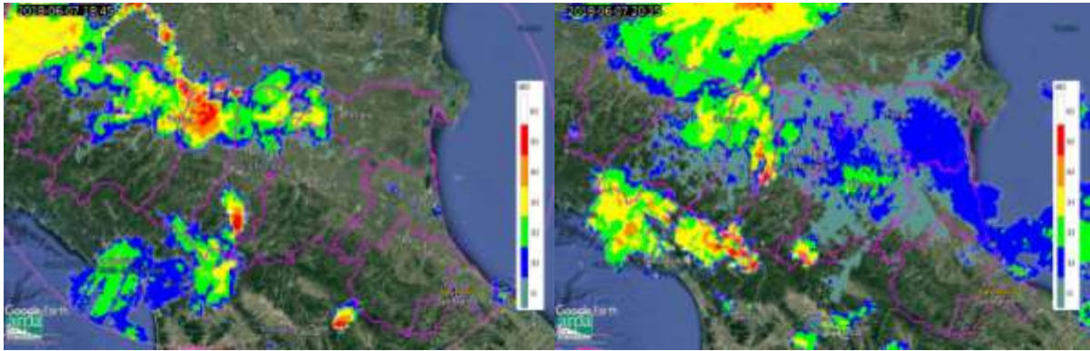
Figura 11. Mappe di riflettività del 07/06/2018 alle 18:45 UTC (a sinistra), alle 20:25 UTC (a destra).
