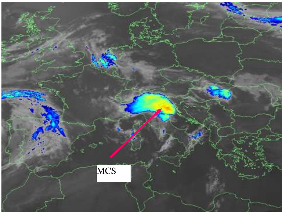
Figura 9. Mappa del prodotto da satellite Enhanced IR del 8/06/2018 ore 04:45 UTC.
