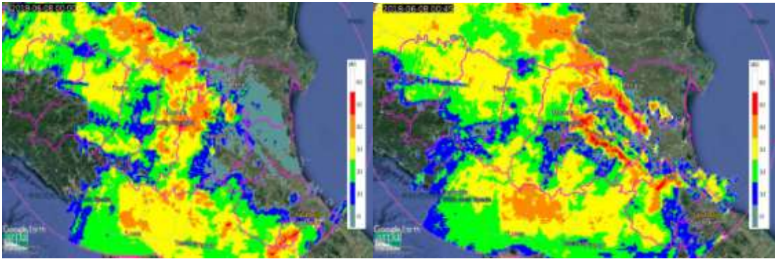
Figura 13. Mappe di riflettività del 08/06/2018 alle 00:00 UTC (a sinistra), alle 00:45 UTC (a destra).
