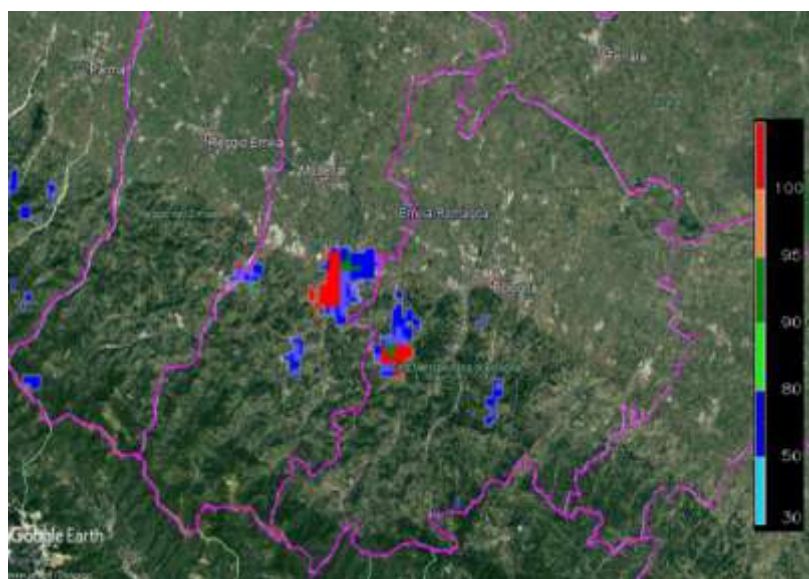
Figura 25. Mappa di riflettività radar (in alto) e di Probability of Hail (in basso) del 07/06/2018 alle 17:40 UTC.
