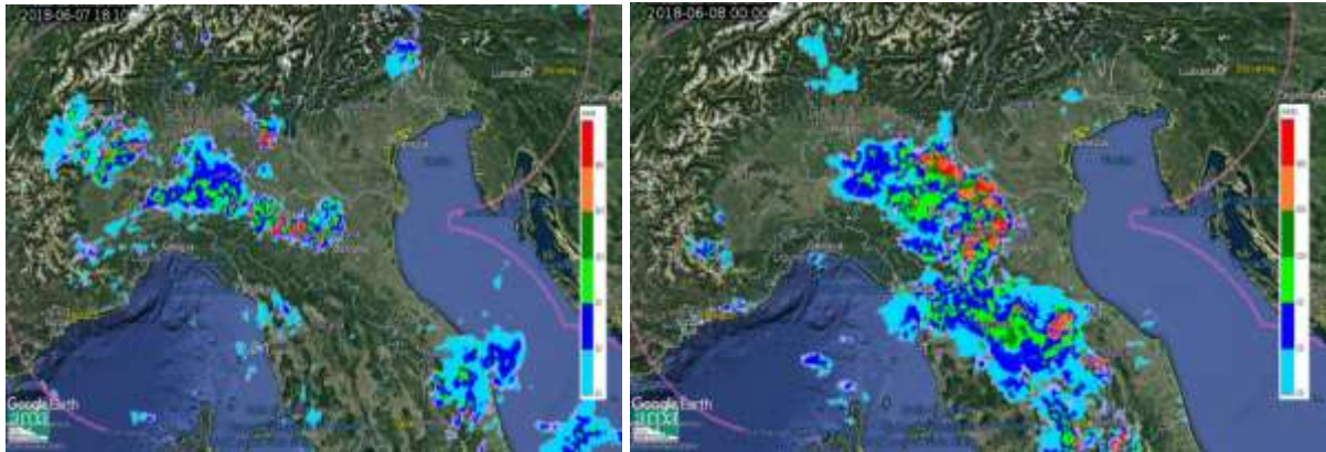
Figura 3. Mappe di precipitazione istantanea stimata dal composito radar nazionale fornito dal Dipartimento di Protezione Civile Nazionale del 07/06/2018 alle 18:10 UTC (a sinistra) e del 08/06/2018 alle 00:00 UTC (a destra).
