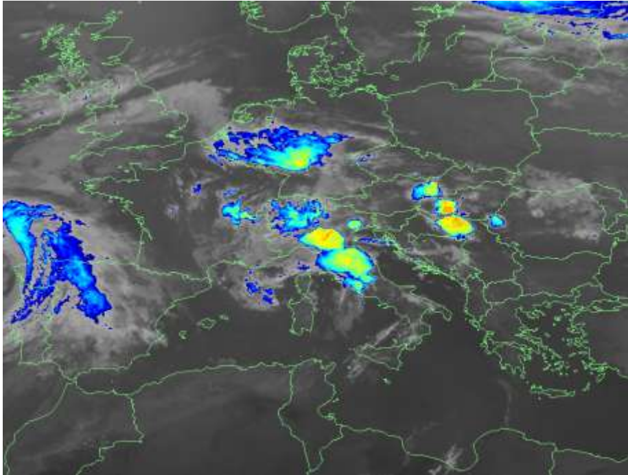
Figura 8. Mappa del prodotto da satellite Enhanced IR del 7/06/2018 ore 22:45 UTC.
