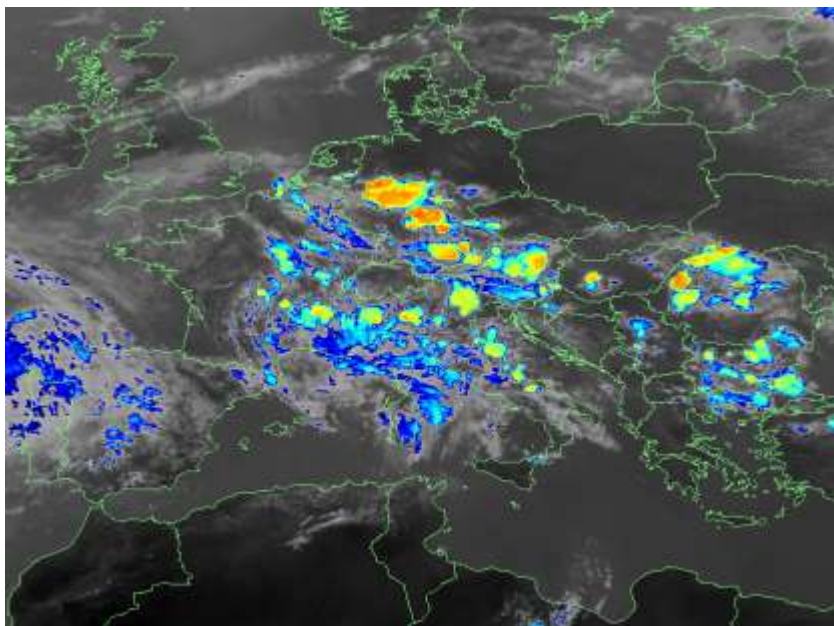
Figura 4. Mappa del prodotto da satellite Enhanced IR del 7/06/2018 ore 15 UTC.
