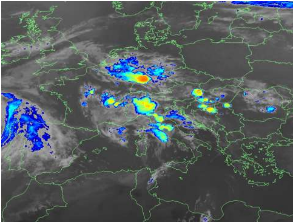
Figura 7. Mappa del prodotto da satellite Enhanced IR del 7/06/2018 ore 21:15 UTC.
