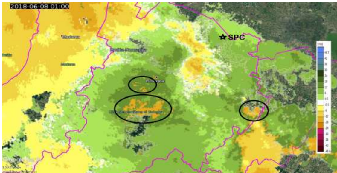
Figura 24. Mappa di velocità radiale del vento doppler da radar del 08/06/2018 alle 01:00UTC.
