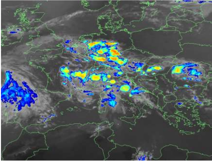
Figura 5. Mappa del prodotto da satellite Enhanced IR del 7/06/2018 ore 18 UTC.
