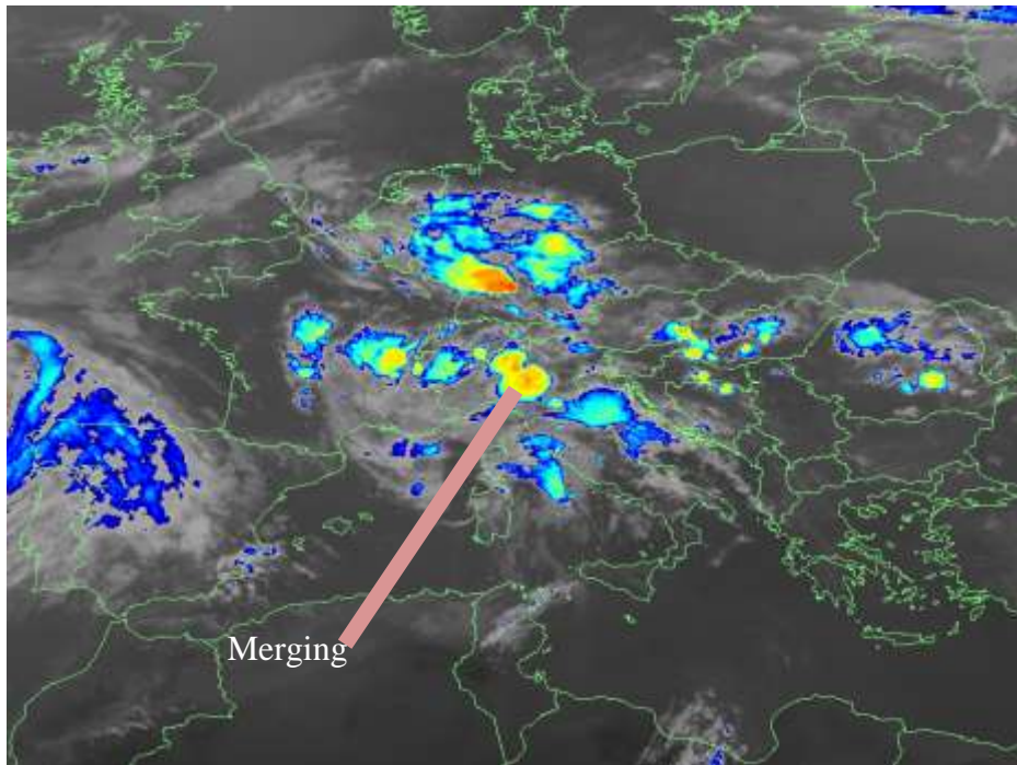
Figura 6. Mappa del prodotto da satellite Enhanced IR del 7/06/2018 ore 19:45 UTC.
