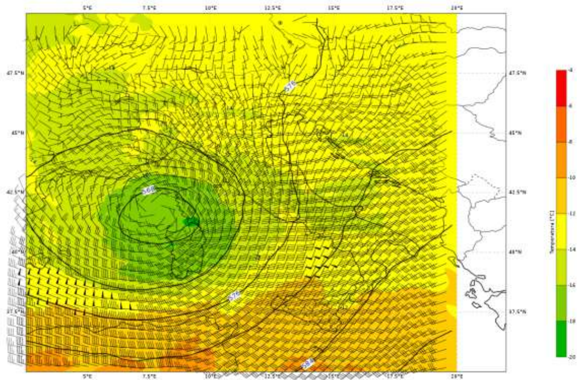
Figura 2. Mappe di analisi (da modello IFS-ECMWF) di geopotenziale, temperatura e vento a 500 hPa del 08/06/2018 alle 00:00 UTC.
