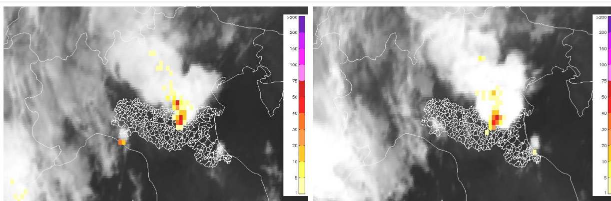
Figura 16. Mappa di fulminazione da rete LAMPINET sovrapposta al canale all'infrarosso del satellite geostazionario Meteosat-11 del 09/08/2018 alle 19:00 UTC (a sinistra) ed alle 19:45 UTC (a destra).
