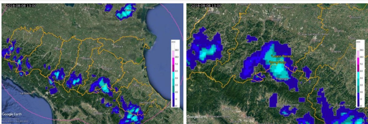
Figura 18. Cumulata di precipitazione oraria stimata da radar dell'08/08/2018 alle 13 UTC (a sinistra) e zoom sulle stazioni, in giallo, che, nell'ora, hanno registrato i valori massimi (a destra).
