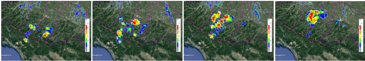
Figura 12. Sequenza di mappe di riflettività del 09/08/2018, da sinistra alle 13:45 UTC, alle 14:15 UTC, alle 14:50 UTC ed alle 15:20 UTC, che mostra l'evoluzione dei sistemi sulle precipitanti sulle province di Modena e Reggio-Emilia.
