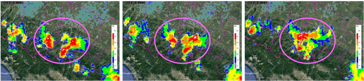
Figura 6. Mappe di riflettività dell'08/08/2018 alle 13:05 UTC (a sinistra), alle 13:20 UTC (al centro) ed alle 13:40 UTC (a destra). In rosa è evidenziata l'unione delle due celle convettive.
