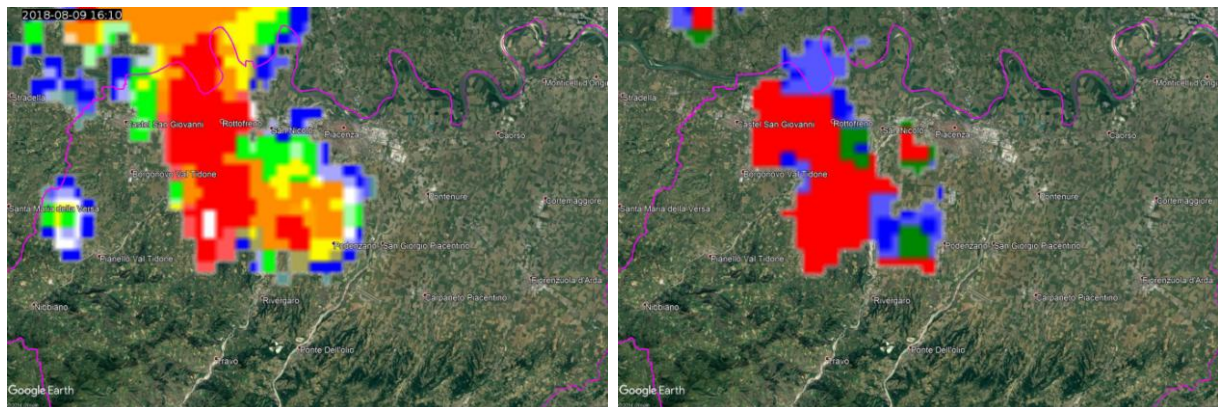
Figura 25. Riflettività osservata alle 16:10 UTC del 09/08/2018 (a sinistra) e corrispondente stima della probabilità di grandine (a destra).
