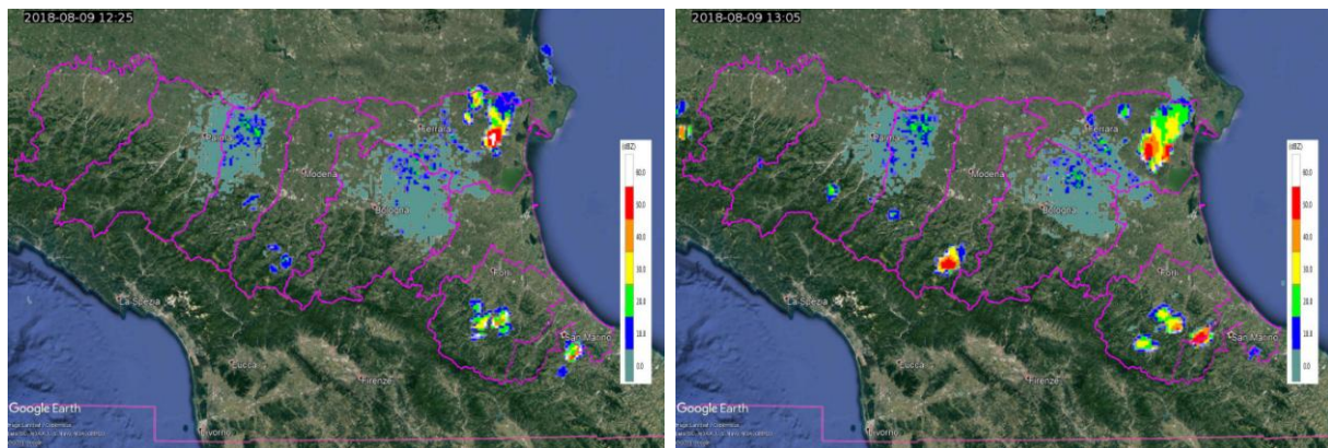
Figura 10. Mappe di riflettività del 09/08/2018 alle 12:25 UTC (a sinistra) ed alle 13:05 UTC (a destra).
