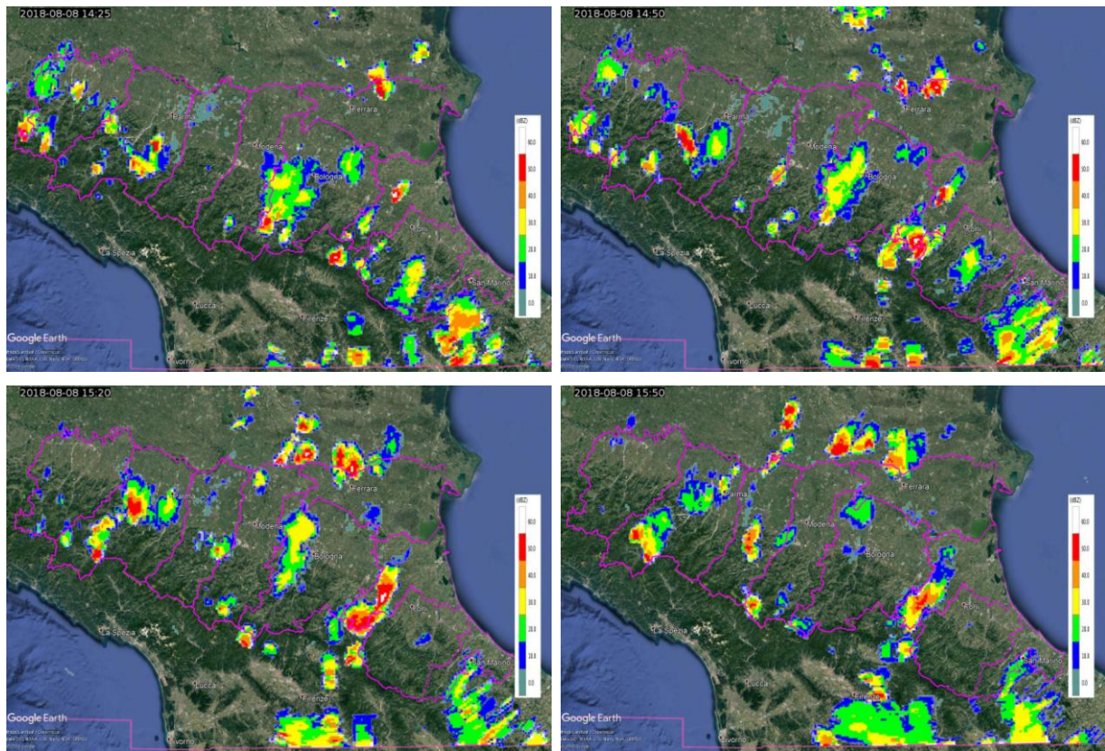
Figura 8. Mappe di riflettività dell'08/08/2018 alle 14:25 UTC (in alto a sinistra), alle 14:50 UTC (in alto a destra), alle 15:20 UTC (in basso a sinistra) ed alle 15:50 UTC (in basso a destra).
