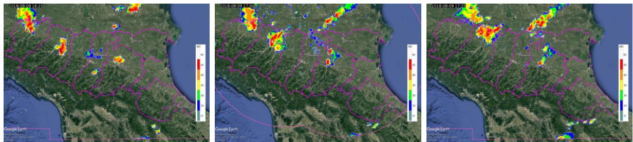
Figura 13. Mappe di riflettività del 09/08/2018 alle 16:25 UTC (a sinistra), alle 17:00 UTC (al centro) ed alle 17:25 UTC (a destra).
