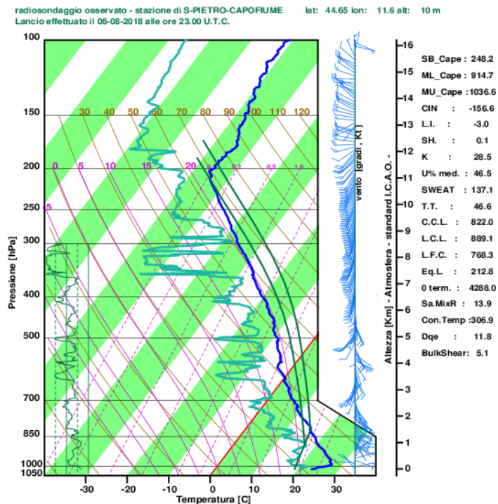
Figura 9. Radiosondaggio termodinamico di San Pietro Capofume (BO) del 09/08/2018 alle 00 UTC
