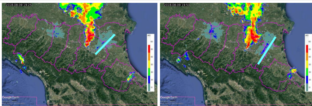
Figura 15. Mappe di riflettività del 09/08/2018 alle 19:25 UTC (a sinistra) ed alle 19:50 UTC (a destra).
