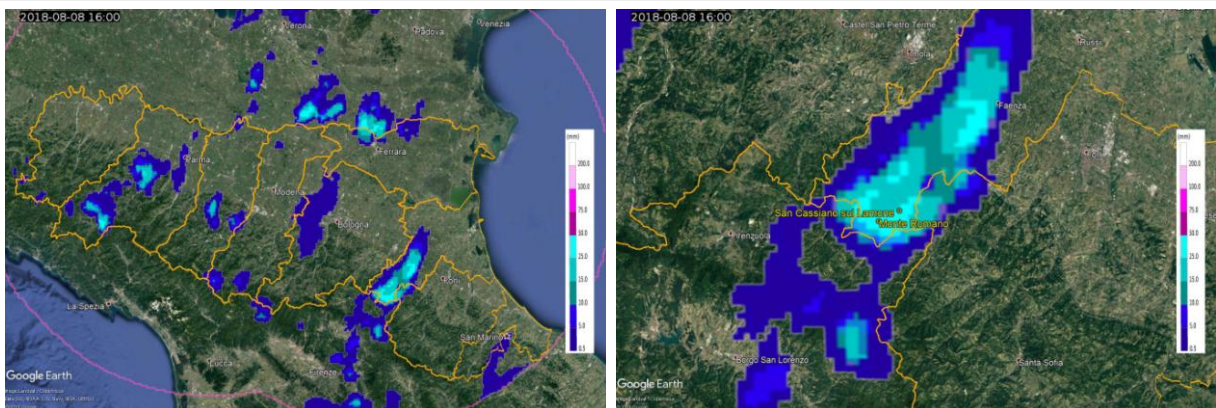
Figura 20. Cumulata di precipitazione oraria stimata da radar dell'08/08/2018 alle 16 UTC (a sinistra) e zoom sulle stazioni, in giallo, che, nell'ora, hanno registrato i valori massimi (a destra).
