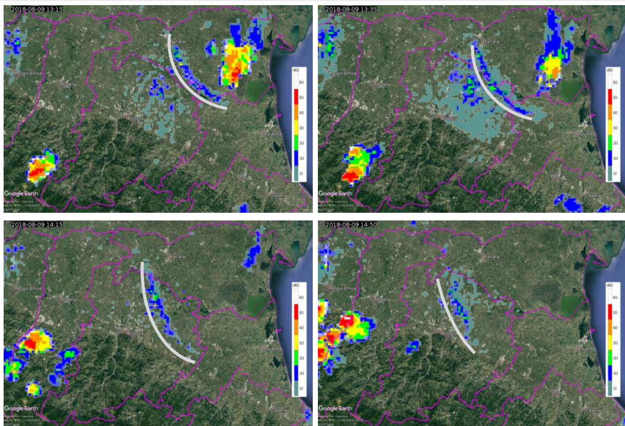
Figura 11. Mappe di riflettività del 09/08/2018 alle 13:15 UTC (in alto a sinistra), alle 13:35 UTC (in alto a destra), alle 14:15 UTC (in basso a sinistra) ed alle 14:50 UTC (in basso a destra). La linea grigia indica lo spostamento del gust front.
