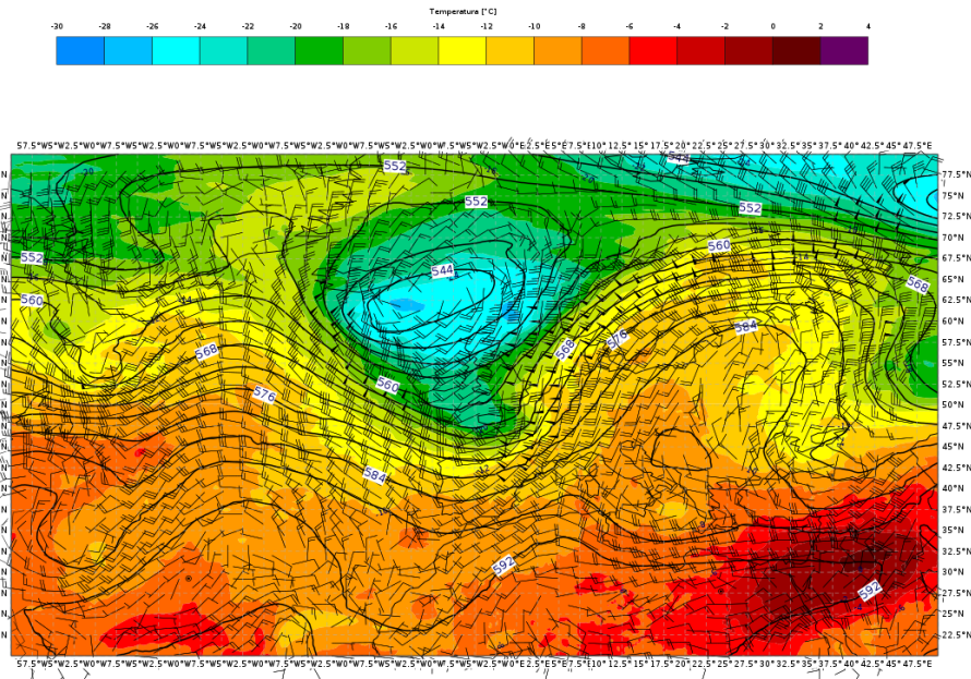
Figura 2. Mapa di analisi (da modello IFS-ECMWF) di geopotenziale, temperatura e vento a 500 hPa del 09/08/2018 alle 12 UTC.
