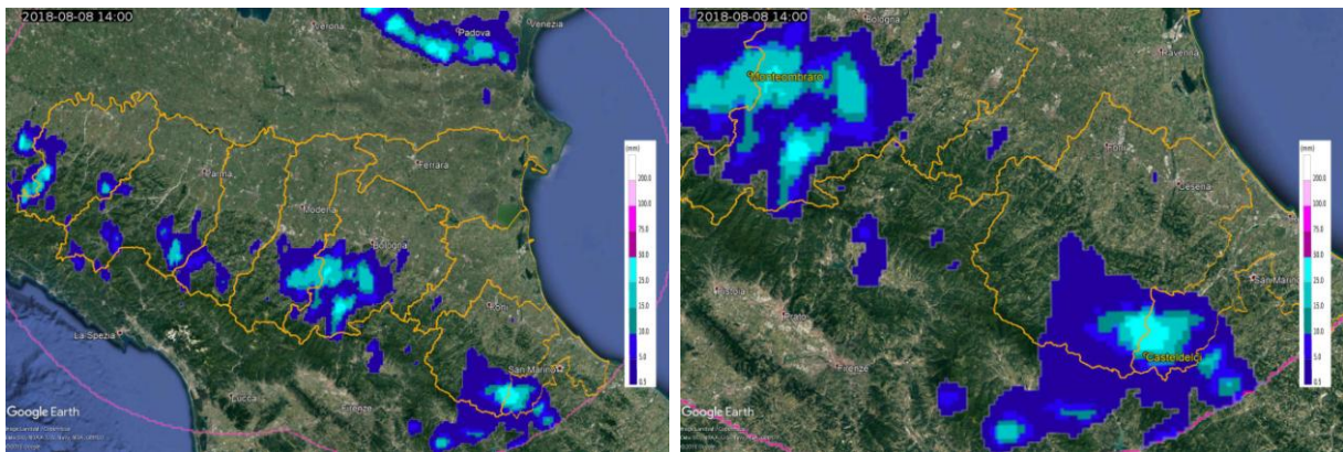
Figura 19. Cumulata di precipitazione oraria stimata da radar dell'08/08/2018 alle 14 UTC (a sinistra) e zoom sulle stazioni, in giallo, che, nell'ora, hanno registrato i valori massimi (a destra).
