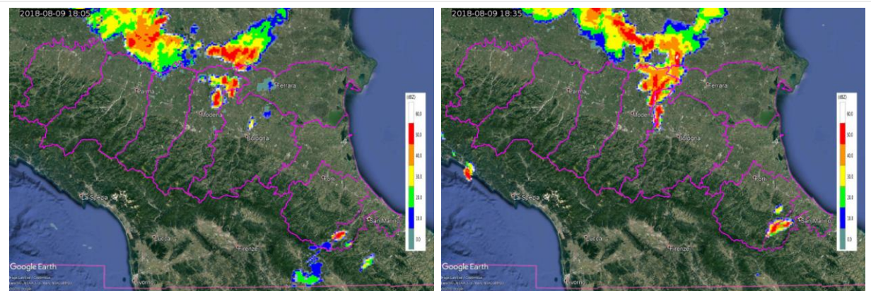
Figura 14. Mappe di riflettività del 09/08/2018 alle 18:05 UTC (a sinistra) ed alle 18:35 UTC (a destra).
