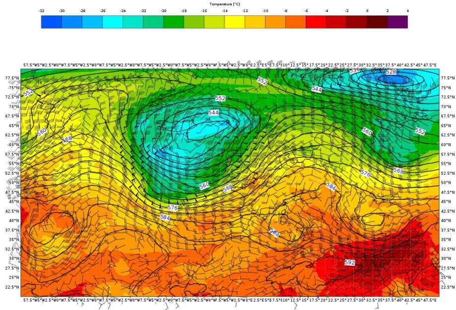
Figura 1. Mapa di analisi (da modello IFS-ECMWF) di geopotenziale, temperatura e vento a 500 hPa dell'08/08/2018 alle 00 UTC.
