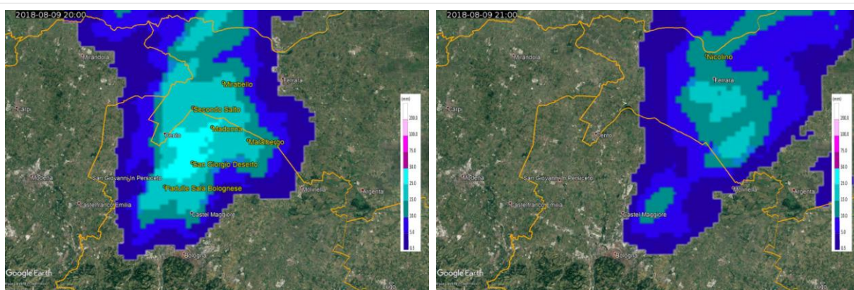
Figura 22. Cumulate di precipitazione oraria stimata da radar del 09/08/2018 alle 20 UTC (a sinistra) ed alle 21 UTC (a destra), centrate sulle stazioni, in giallo, che hanno registrato i valori massimi nell'ora e nei 15 minuti.
