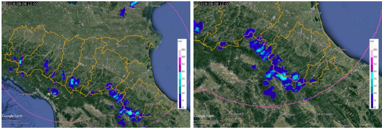
Figura 17. Cumulata di precipitazione oraria stimata da radar dell'08/08/2018 alle 12 UTC (a sinistra) e zoom sulla stazione di Lama (FC) che, nell'ora, ha registrato il valore massimo (a destra).
