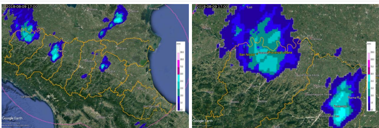
Figura 21. Cumulate di precipitazione oraria stimata da radar del 09/08/2018 alle 17 UTC (a sinistra) e zoom sulle stazioni, in giallo, che, nell'ora, hanno registrato i valori massimi (a destra).
