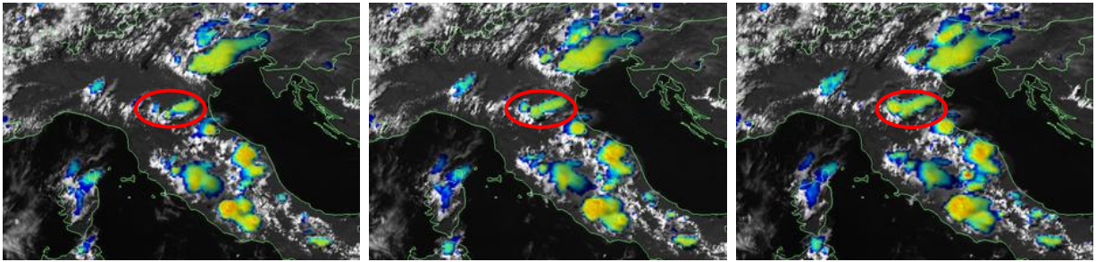
Figura 5. Sequenza di immagini del prodotto Enhanced Infrared sul canale del visibile ad alta risoluzione HRV del satellite geostazionario Meteosat-11 dell'08/08/2018 alle 13:00 UTC (a sinistra), alle 13:15 UTC (al centro) ed alle 13:30 UTC (a destra). In rosso è evidenziata l'area su cui avviene l'evoluzione e la conseguente unione delle due celle convettive.
