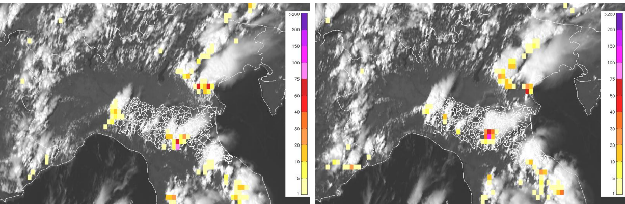
Figura 7. Mappa di fulminazione da rete LAMPINET sovrapposta al canale del visibile ad alta risoluzione HRV del satellite geostazionario Meteosat-11 dell'08/08/2018 alle 13:15 UTC (a sinistra) ed alle 13:45 UTC (a destra).
