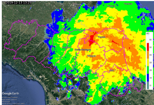
Figura 16: Mappa di riflettività del composito radar del 13/12/2019 alle 13:25 UTC.
