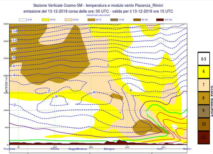
Figura 15: Sezione verticale tra Piacenza e Rimini, dal modello COSMO a 5km, di temperatura e modulo del vento del 13/12/2019 alle 15 UTC.
