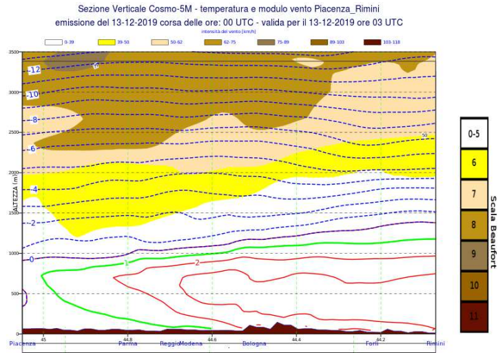
Figura 4: Sezione verticale tra Piacenza e Rimini, dal modello COSMO a 5km, di temperatura e velocità del vento del 13/12/2019 alle 03 UTC.
