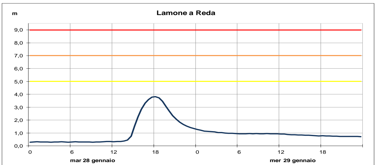
Figura 16: Andamento dei livelli idrometrici nelle sezioni vallive più significative del fiume Lamone e del suo affluente Marzeno (ora solare - dati validati).
