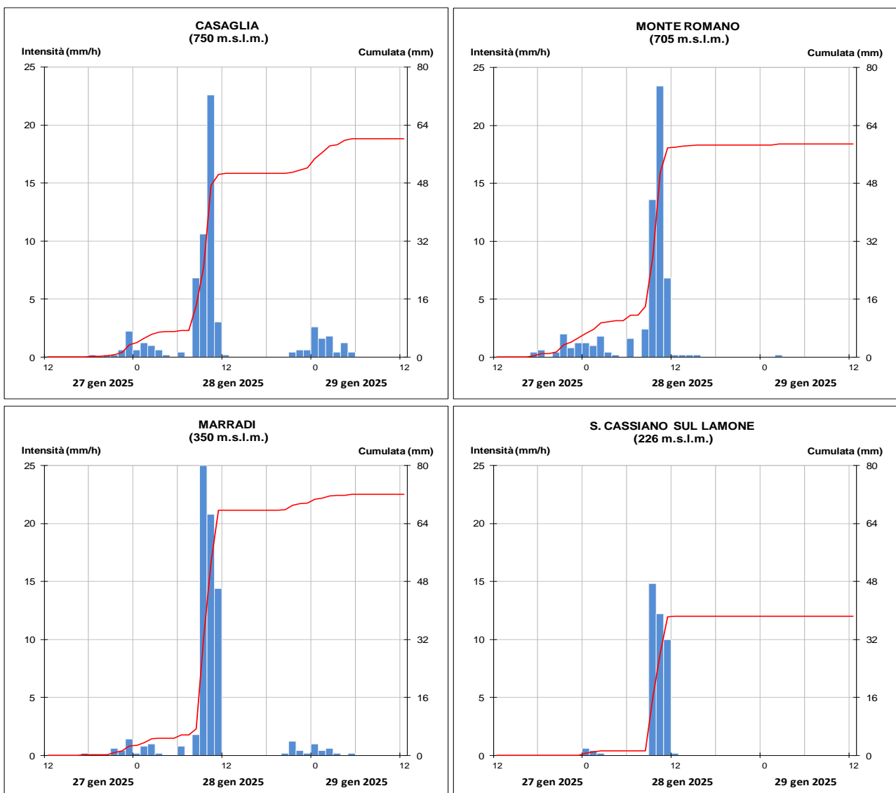
Figura 14: Andamento delle precipitazioni orarie e cumulate più significative dell'evento del 27-28 gennaio, registrate dai pluviometri del bacino del Lamone (ora solare - dati validati.)
