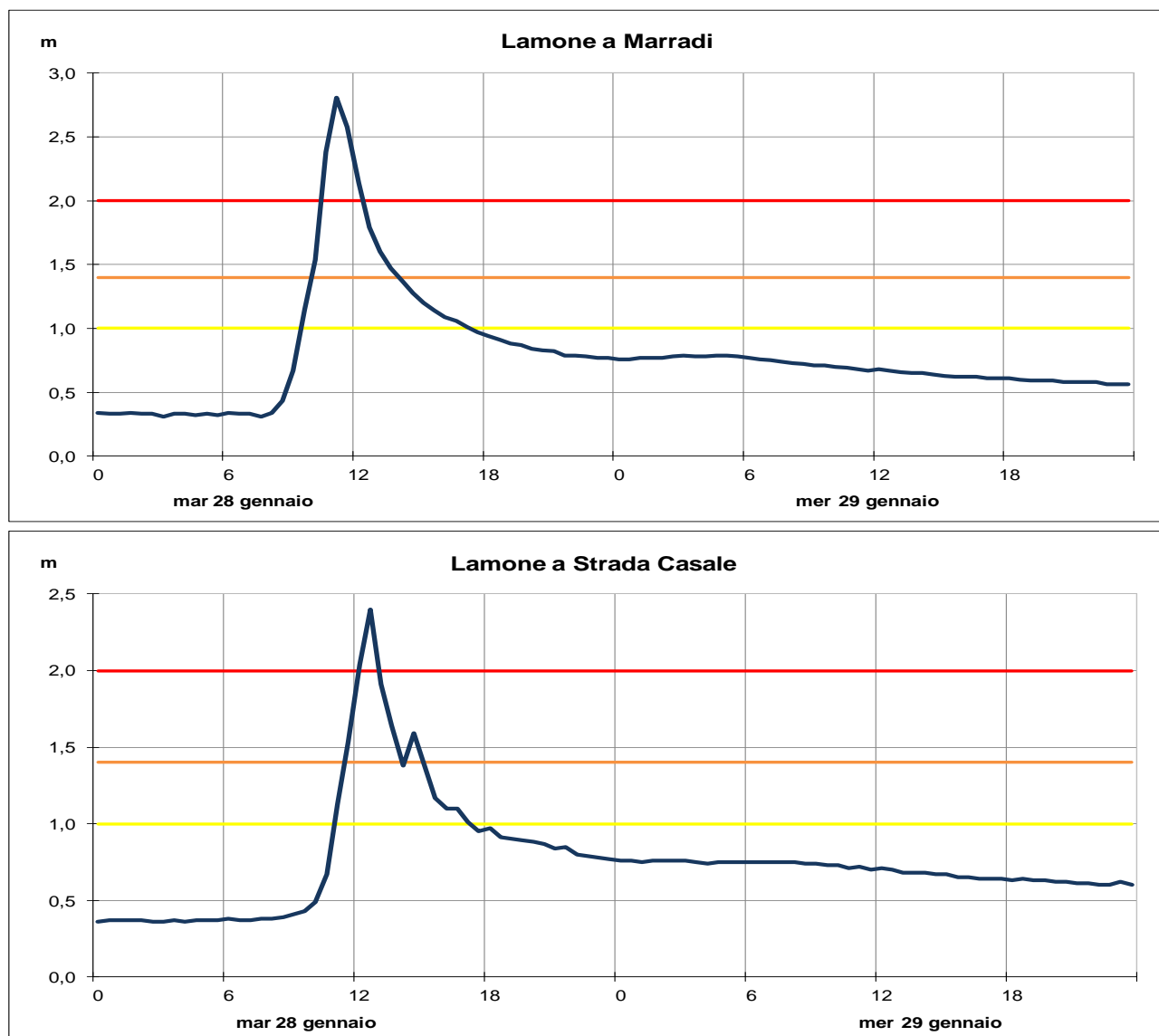
Figura 15: Andamento dei livelli idrometrici nelle sezioni montane più significative del fiume Lamone (ora solare - dati validati).
